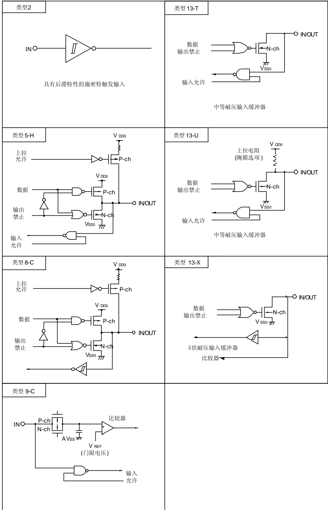
图 3-1. 引脚 I/O 电路
